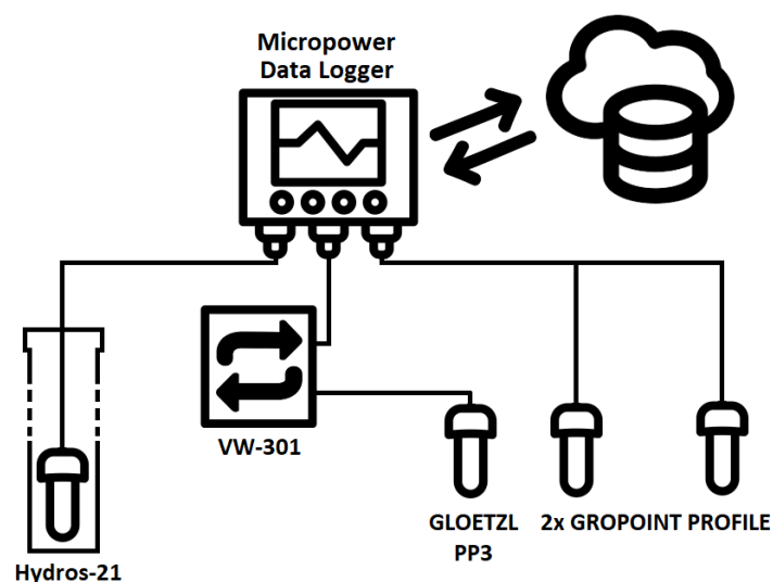
Rys. 1. Architektura systemu monitorowania stanu wału przeciwpowodziowego
