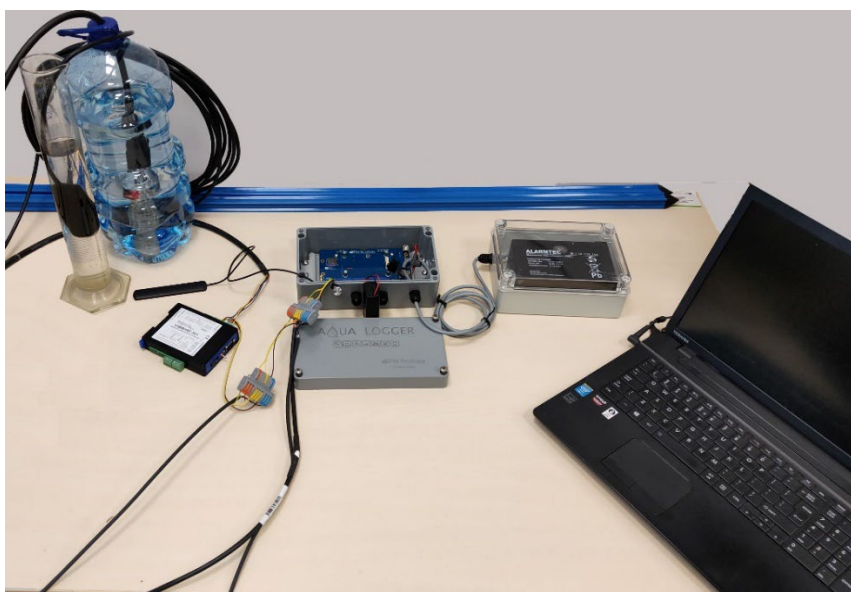
Rys. 2. System pomiarowy w warunkach laboratoryjnych Fig. 2. Measurement system in laboratory conditions
