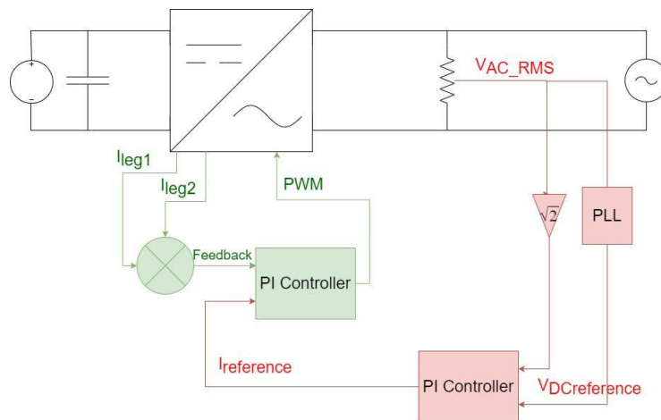
Fig. 4. Loops of voltage and current control Rys. 4. Pętle sterowania napięciem i prędem
