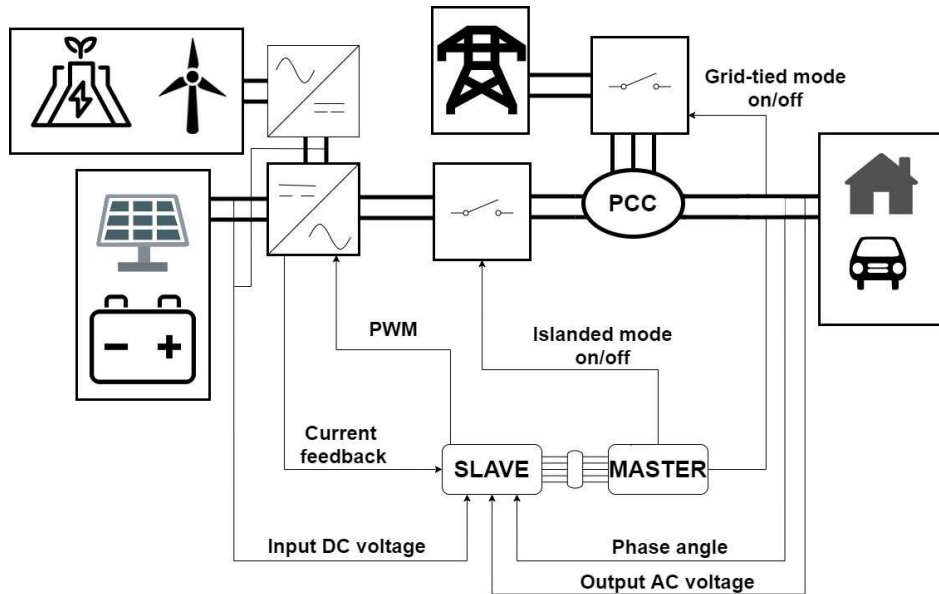
Fig. 2. Diagram of an example Micro Grid Rys. 2. Schemat blokowy przykładowej Mikrosieci
