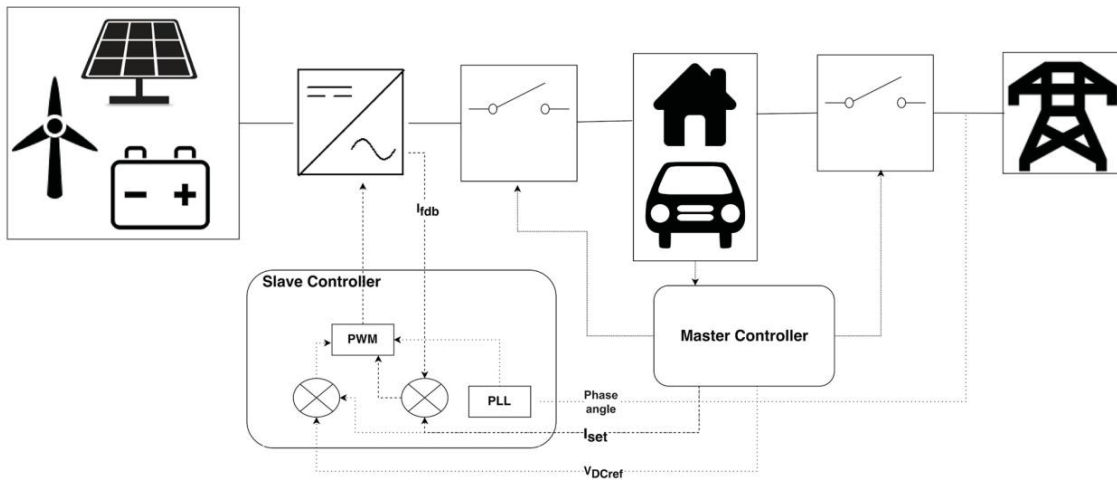
Fig. 1. Diagram of an example Micro Grid Rys. 1. Schemat blokowy przykładowej Mikrosieci
